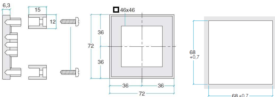
Tafelausschnitt
