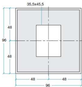
96x96 / 2TE
