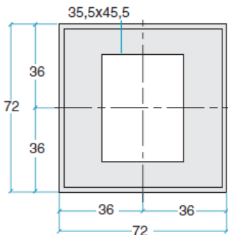
72x72 / 2TE
