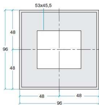
96x96 / 3TE
