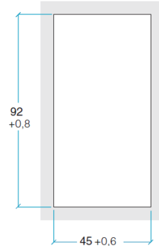
Tafelausschnitt
