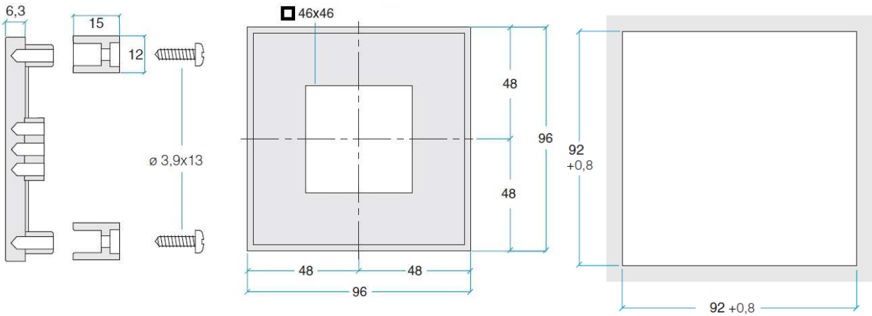
Tafelausschnitt
